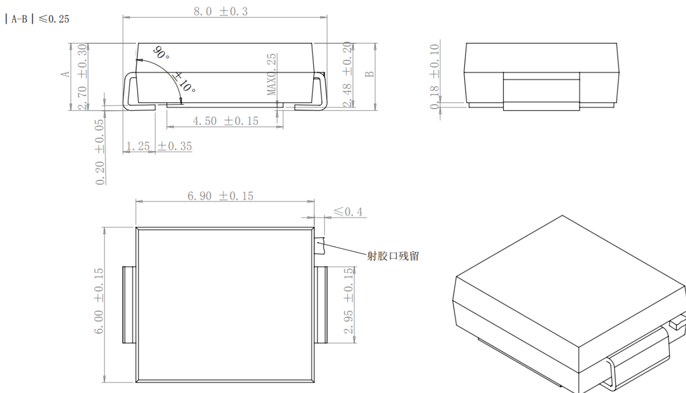
DO-214AB(smc)
